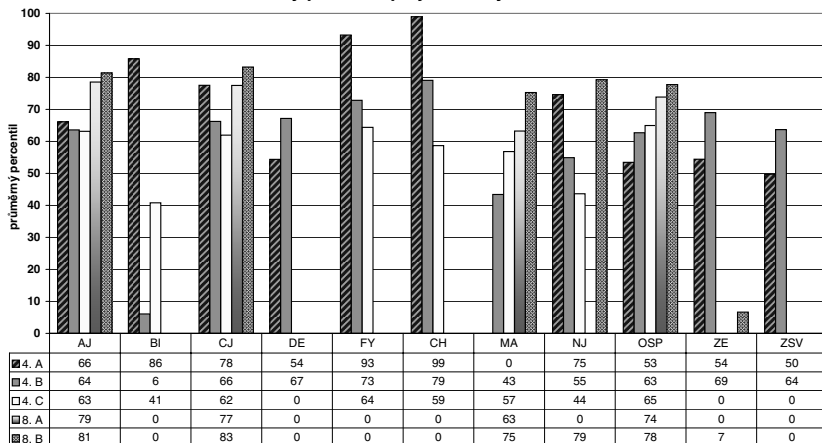
Průměrný percentil po jednotlivých třídách
